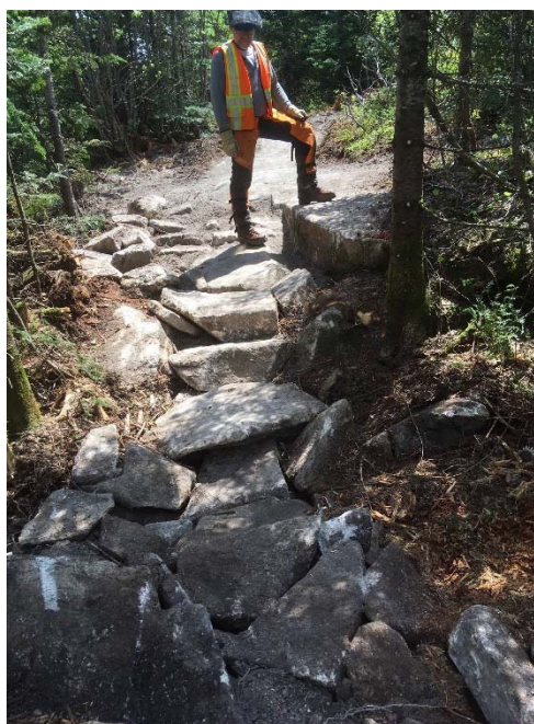
Figure 6 : Marches du Sentier des Géants en construction par l'équipe d'Aménagements Sentiers Verts (ASV) à l'été 2019.
